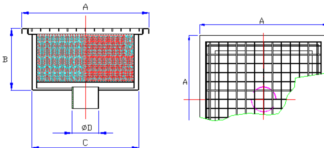
SCHEMA MONTAGGIO A PAVIMENTO DI UN CHIUSINO ICxP GV CON SCARICO VERTICALE
