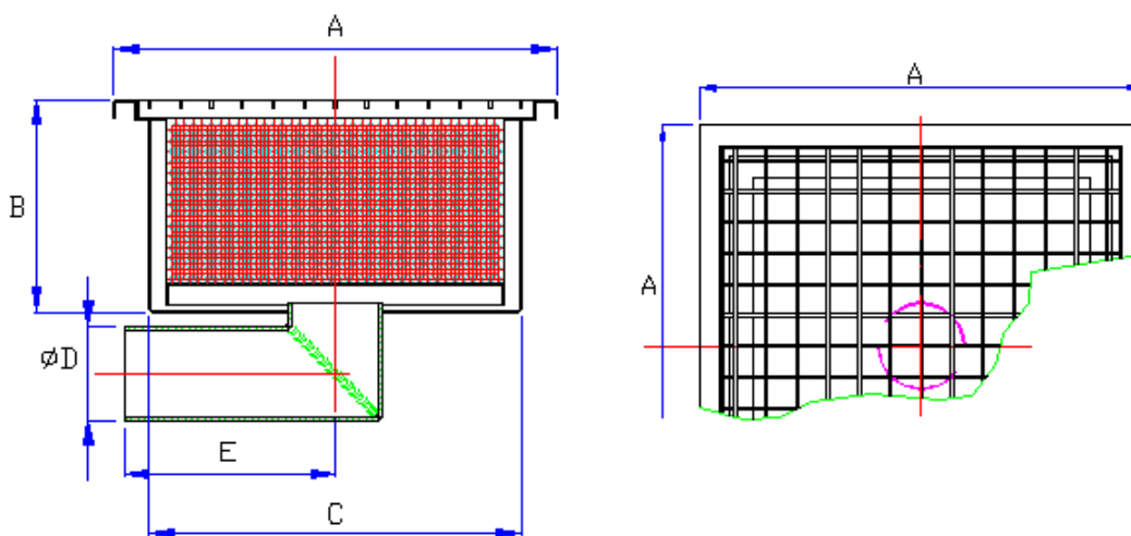
DISEGNI TECNICI DEL CHIUSINO ICxP GL CON SCARICO LATERALE
