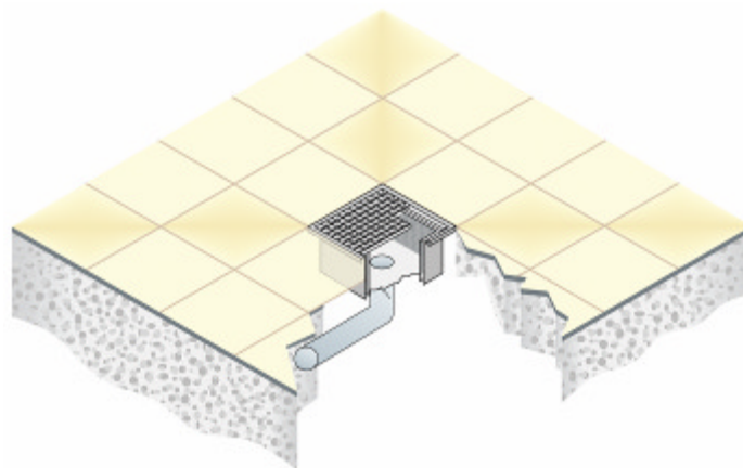
SCHEMA MONTAGGIO A PAVIMENTO DI UN CHIUSINO ICxP GL CON SCARICO LATERALE
