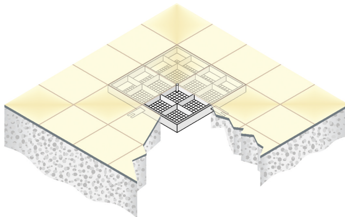
SCHEMA MONTAGGIO A PAVIMENTO DI UN CHIUSINO ICxP B
