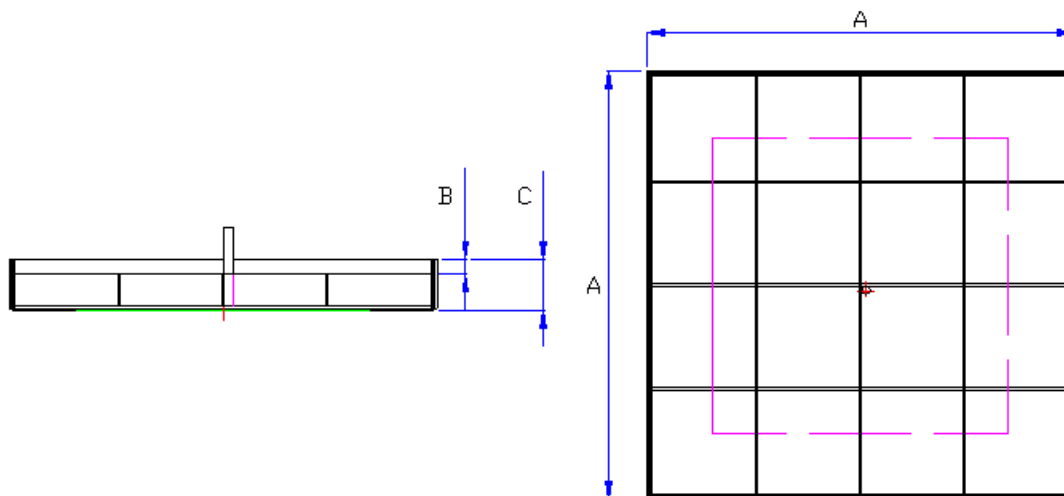
DISEGNI TECNICI DEL CHIUSINO ICxP B
